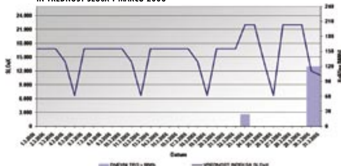
GIBANJE CEN IN KOLIČIN DODELJENIH ČEZMEJNIH PRENOSNIH ZMOGLJIVOSTI V SMERI IZ HRVAŠKE V SLOVENIJO V MARCU 2006
